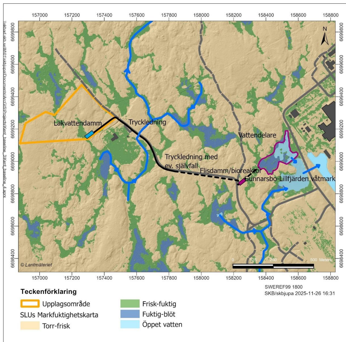
Figur 4. Planerat system för kväverening.
