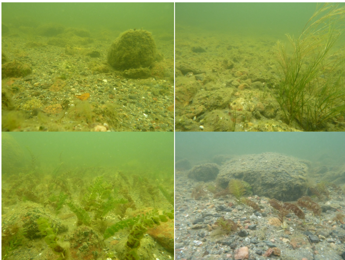
Bild 8:2. Transekt LFM001078. Öv, Öh: Sparsamt med växtlighet trots det ringa djupet ca 1 m. Nv: Ålnate i ett tätare litet bestånd. Nh: Ytnära botten med spridda ålnate och lite fintrådig på blocken.
