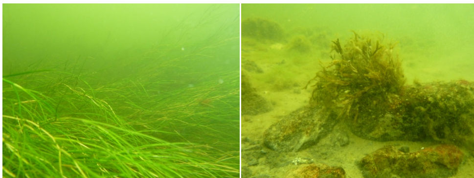
Figur 2. Vegetation på grunda havsbottnar vid SFR. V: Borstnate i frodigt bestånd. H: Småltång på blockig sandbotten.
