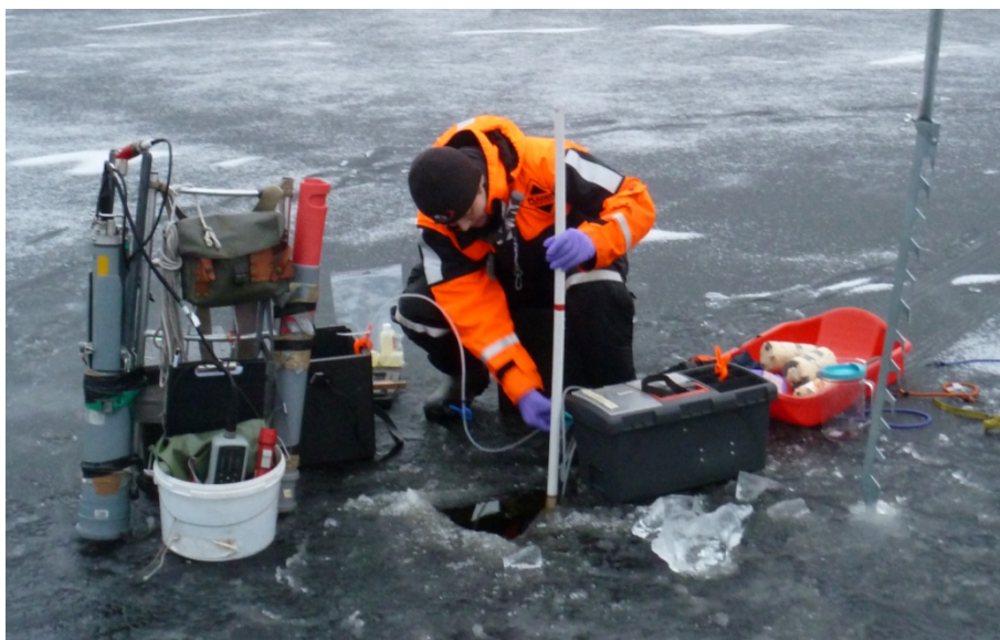
Figur 22. Vattenkemiska provtagningar och mätningar utförs året runt vid övervakningsstationen (PFM000062) i Asphällsfjärden.
