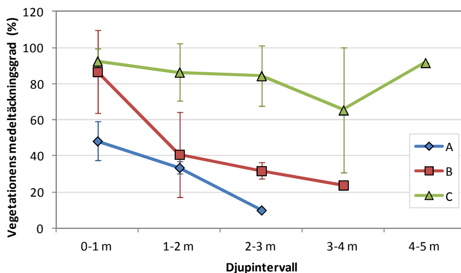
Figur 9. Vegetationens medeltäckningsgrad ( \pm standardavvikelse) i enmetersdjupintervall beräknat per delområde A, B och C.
