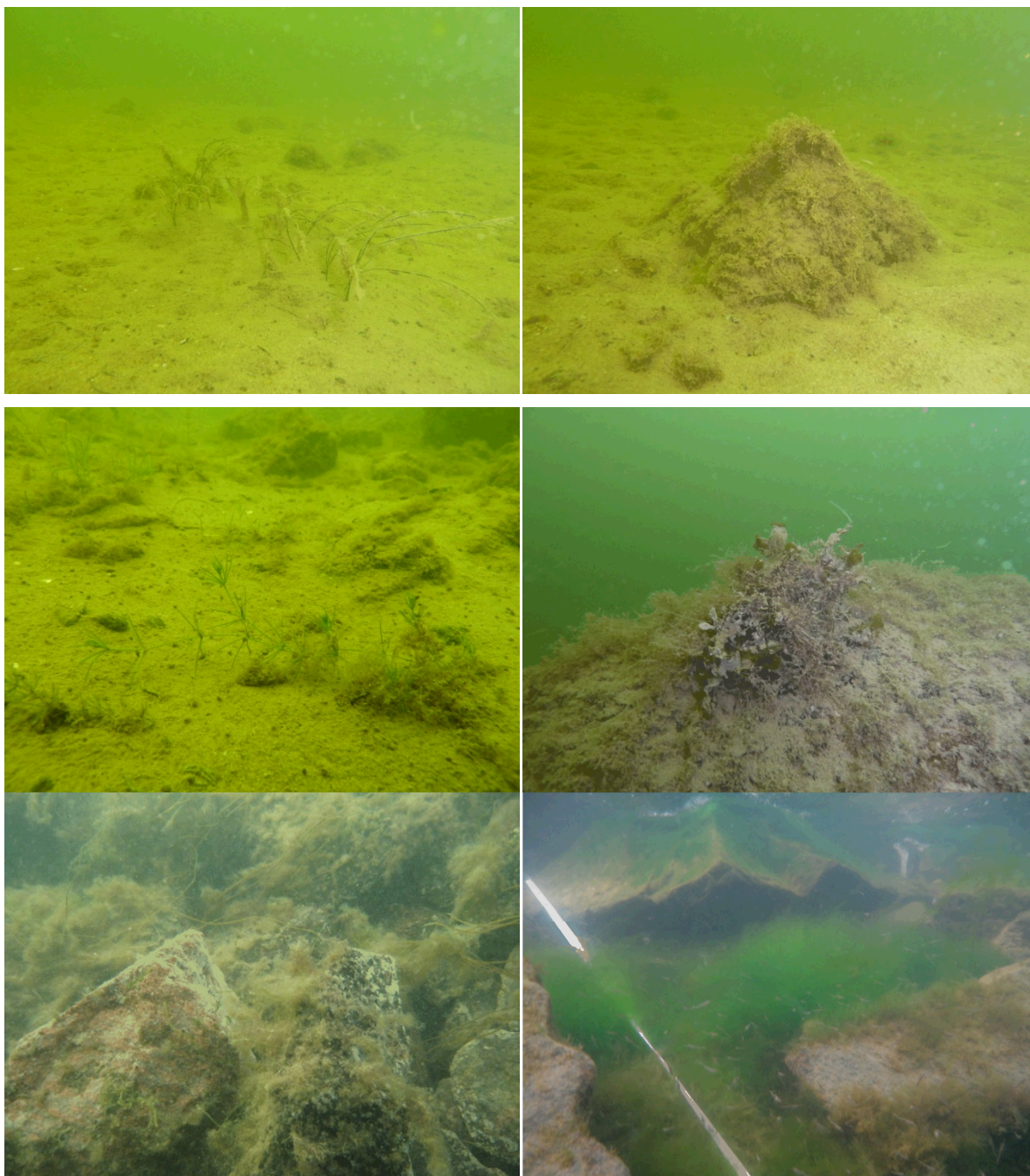
Bild 8:7. Transekt LFM001083. Öv: Spridda borstnate på 3-4 m djup. Öh: Block med fintrådiga alger 3-4 m djupt. Mv: Enstaka kransalger på sandig och stenig botten. Mh: En liten smaltångsruska med mycket påväxt. Nv: Grunda block med fintrådiga alger. Nh: Ytnära block med tarmalger och grönslick.
