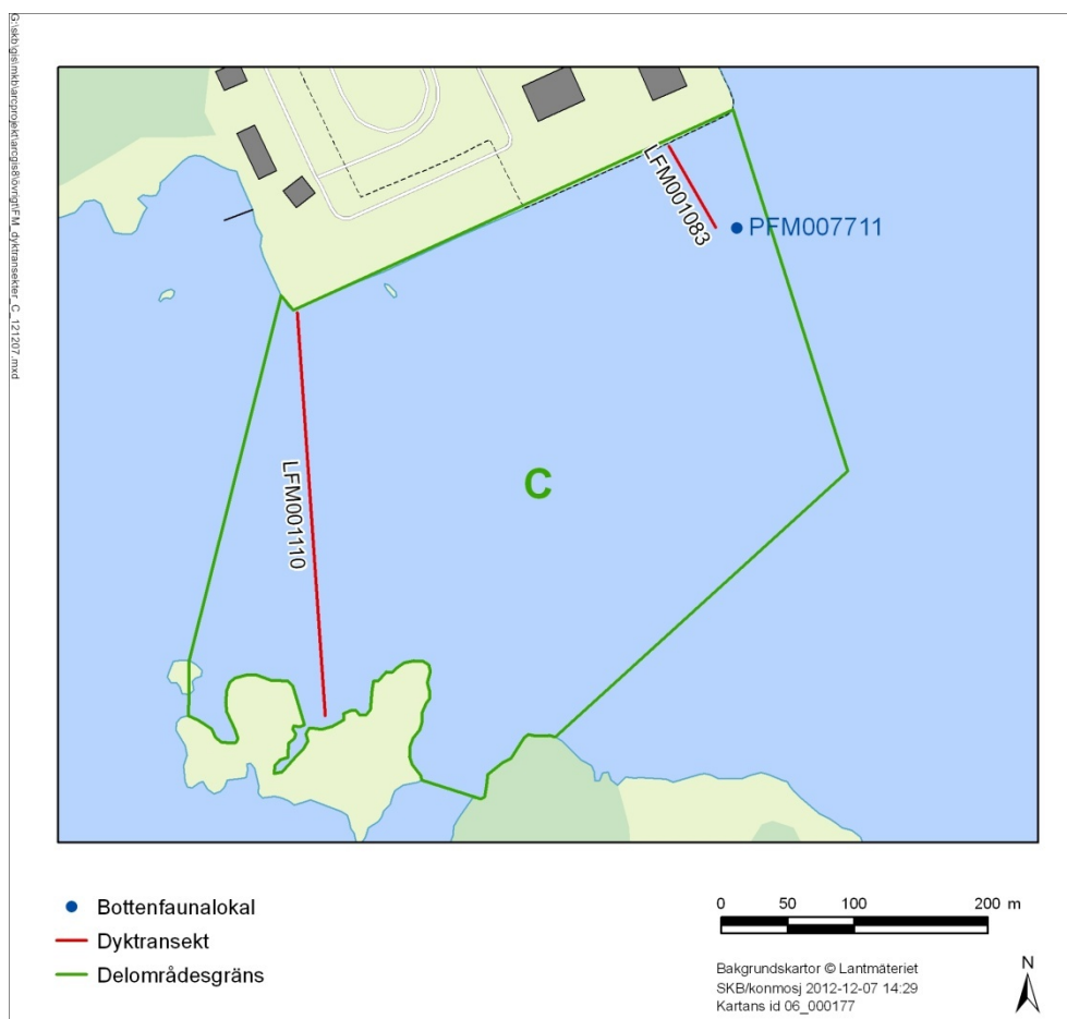
Figur 4d. Delområde C. De två inventerade transekterna LFM001083 samt LFM001110 (referenstranssekt) är markerade. I kartan visas även bottenfaunalokalen PFM007711.
