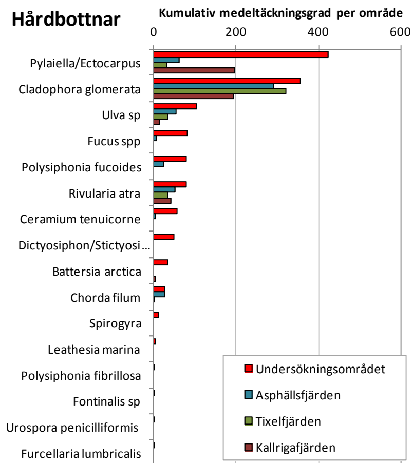
Figur 18. Artsammansättning på hårdbottnar. Medeltäckningsgraden beräknad per enmetersdjupintervall summerad per område som ett översiktligt mått på förekomst och utbredning i respektive område. Undersökningsområdet inkluderar ej transekt LFM1110 och i Asphällsfjärden ej fem transekter i strömfåran (LFM660, LFM661, LFM662, LFM663 och LFM675).
