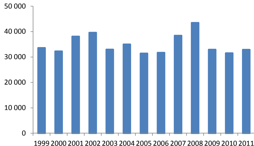
Figur 10. Modellberäknad totalkvävebelastning för Öregrundsgrepen 1999–2011 (SMHI 2013).
