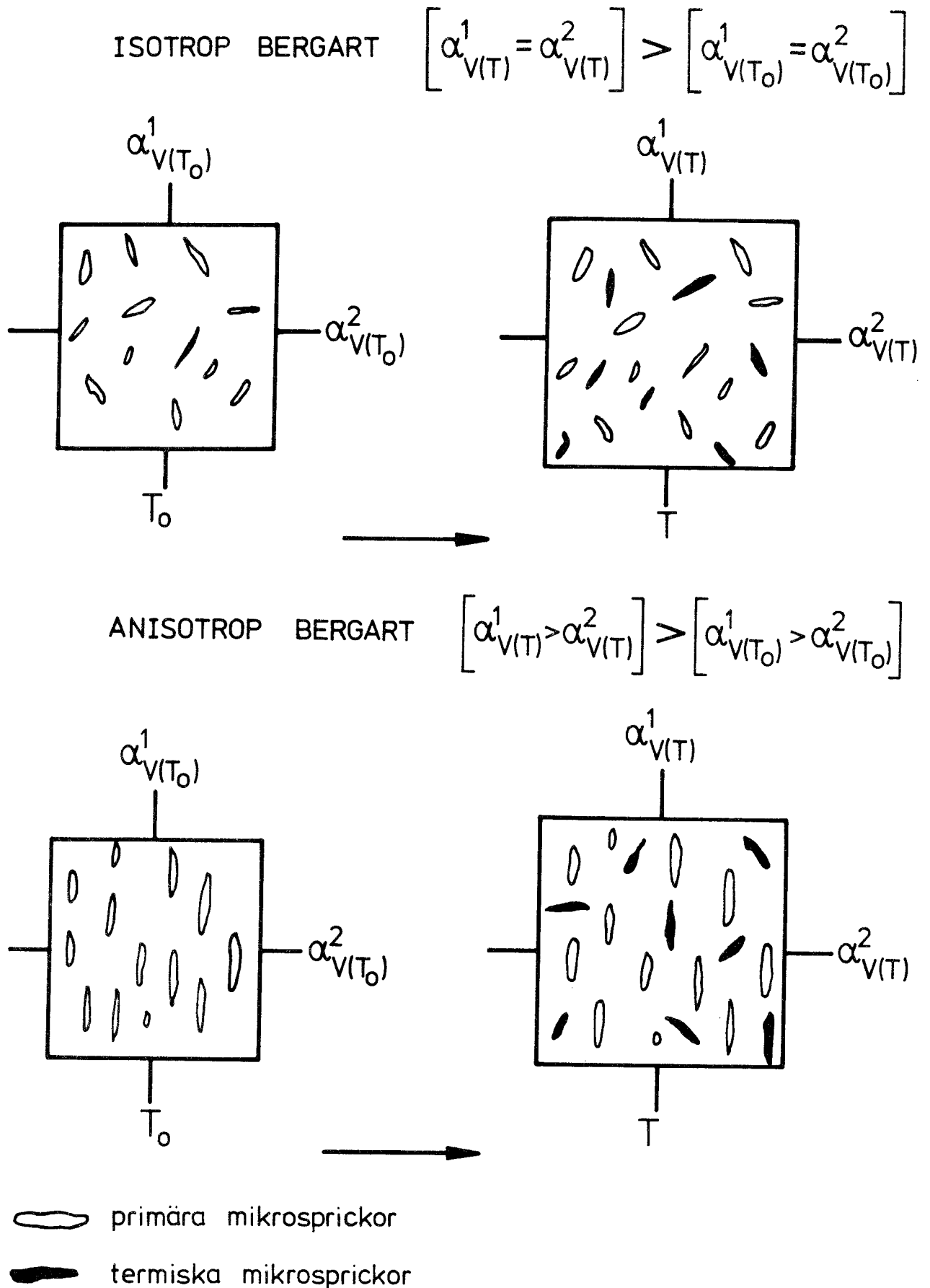
Fig 5 Mikrosprickornas bildning och volymutvidgningskoefficientens variation med ökad temperatur för isotrop och anisotrop bergart
