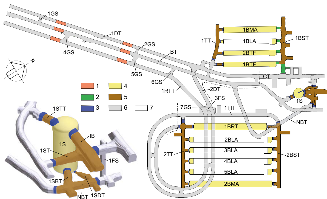
Figur B2-1. Figuren visar pluggarnas position med olika färgsättningar. Brun färg: bentonit (de täta sektionerna). Blå färg: betongplugg. Grön färg: jorddammsplugg. Orange färg: pluggar i nedfartstunnlar. Gul färg: återfyllnadsmaterial i bergsalarna.
