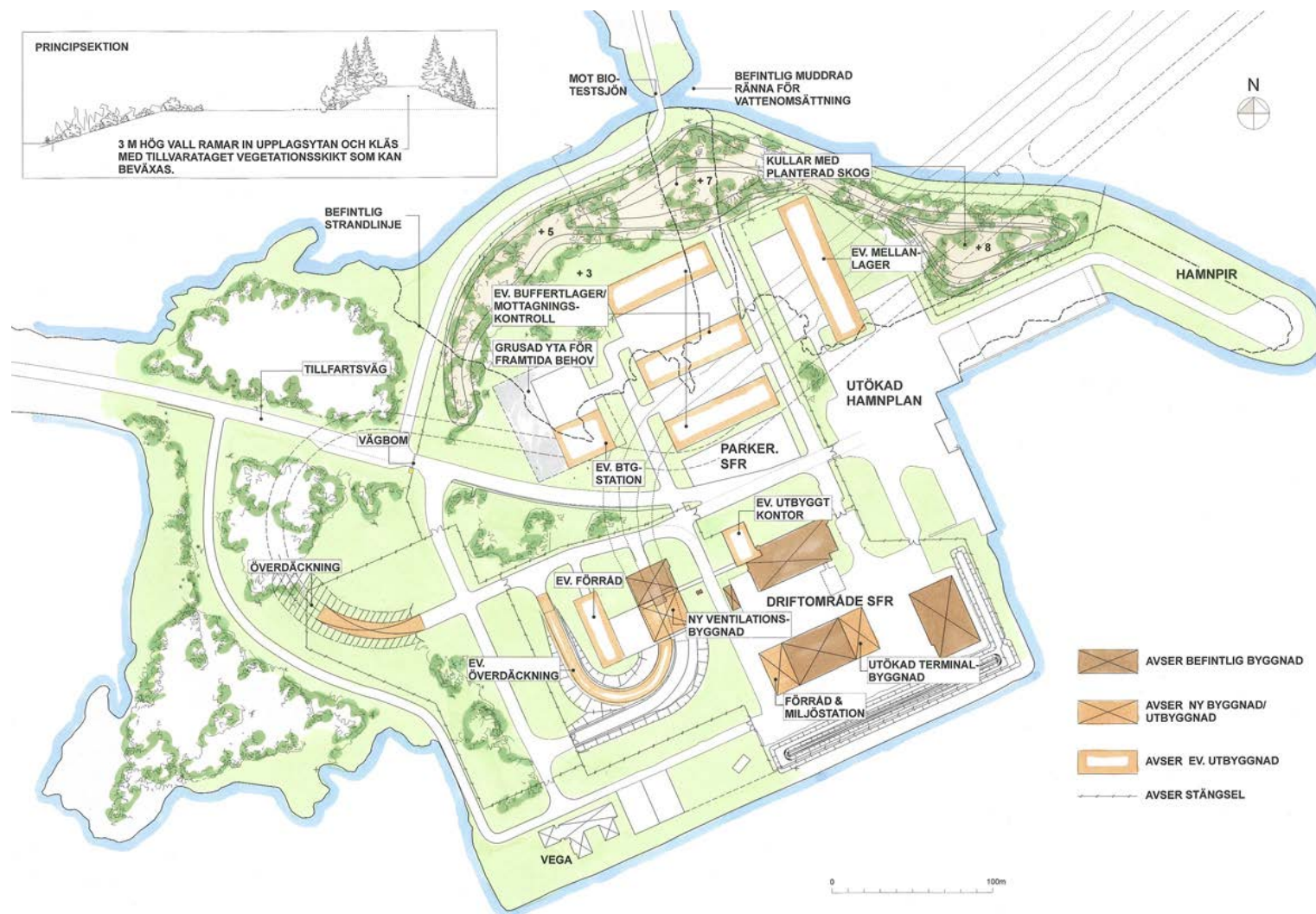
Figur B1-1. Situationsplan för driftområde.
