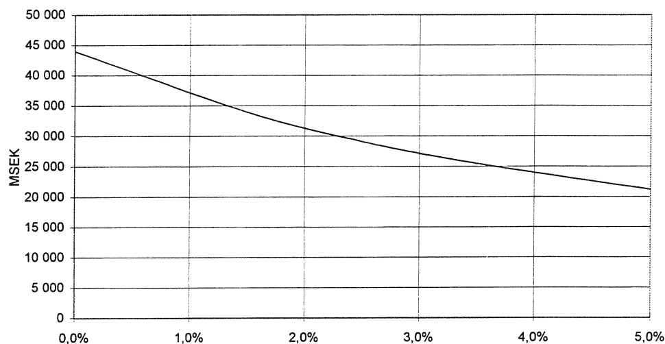
Figur 4.3 Totala framtida kostnader enligt finansieringslagen som funktion av real kalkylränta. Drift av samtliga reaktorer 25 år eller minst t o m 1998. Prisnivå januari 1997
