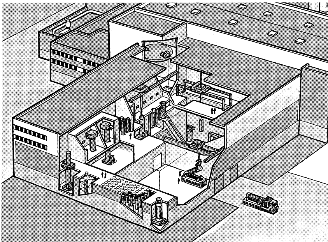
Figur 2.7 Inkapslingsanläggning för använt bränsle
