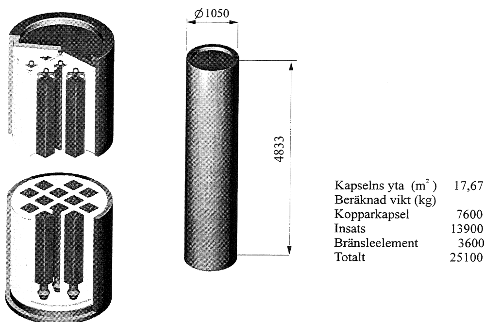
Figur 2.6 Kopparkapsel med inre stålbehållare
