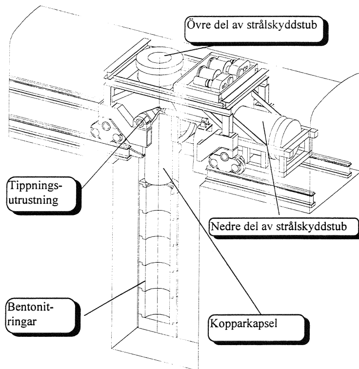
Figur 2.3 Skiss av maskinen för nedsättning av kapsel
