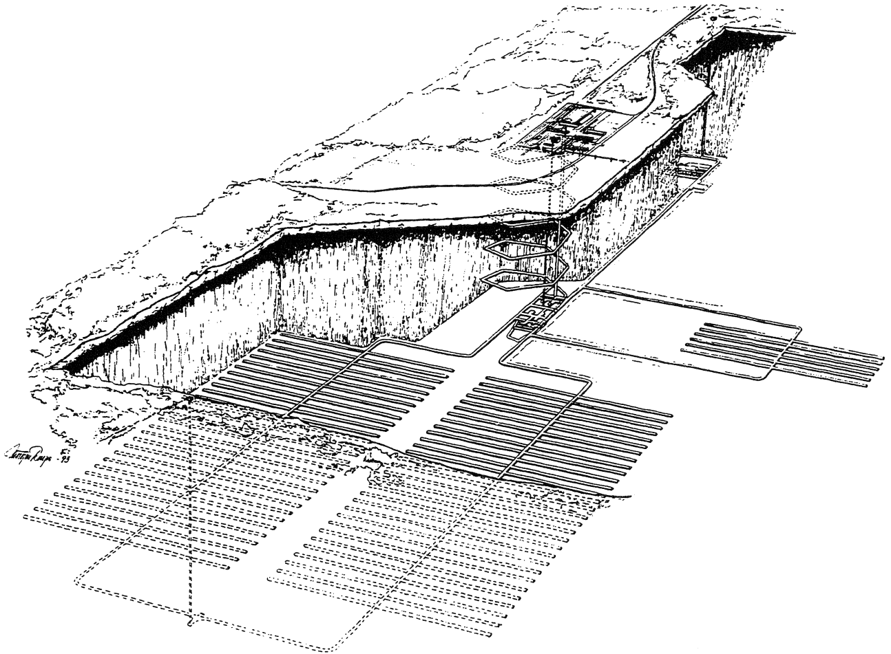
Figur 2.9 Djupförvar - översikt
